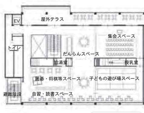
2階平面図
